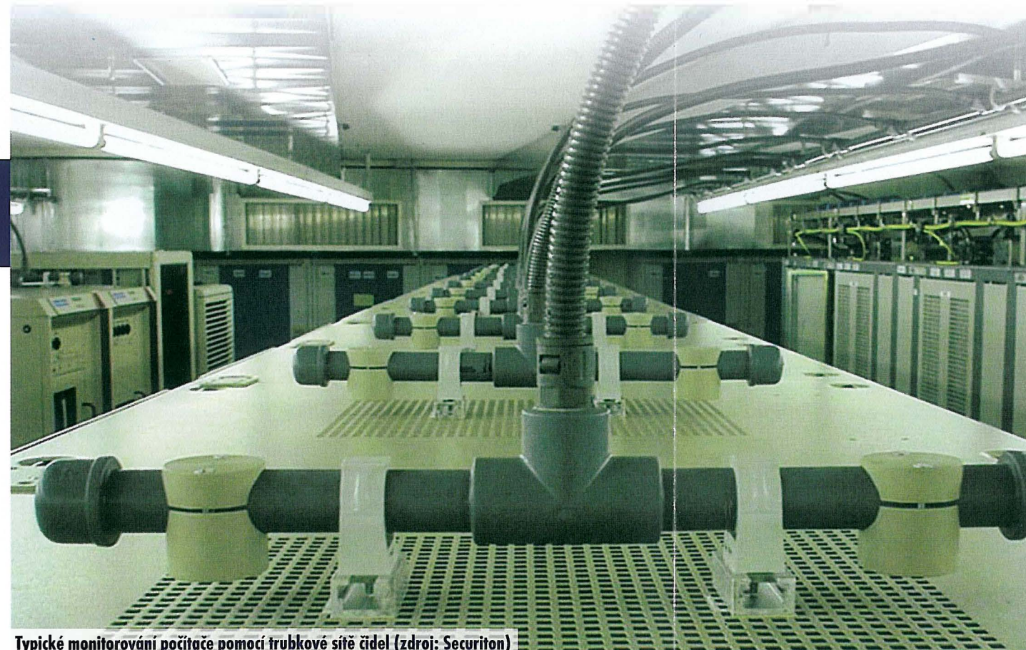
Typické monitorování počítače pomocí trubkové sítě čidel (zdroj: Securiton)
