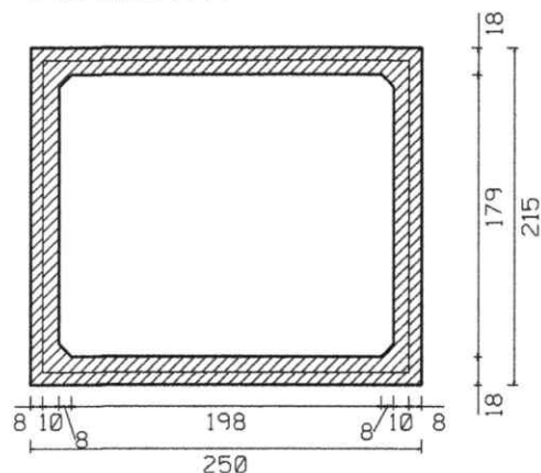
POHLED A-A'
