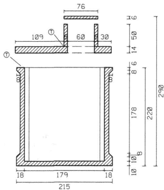
ŘEZ B-B'
