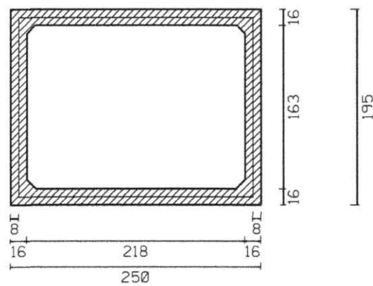
ŘEZ C-C'
