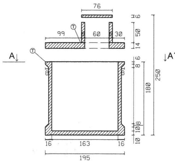
ŘEZ C-C'
