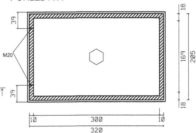
POHLED A-A'
