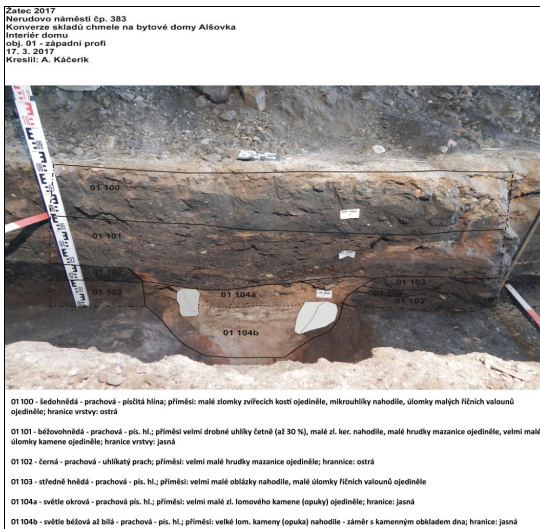
Obr. 06. Interpretovaná pozitivní nálezová situace, příčný řez výplní zahloubeného archeologického objektu do staršího kulturního souvrství z raného středověku; foto a kresba A. Káčerik.
