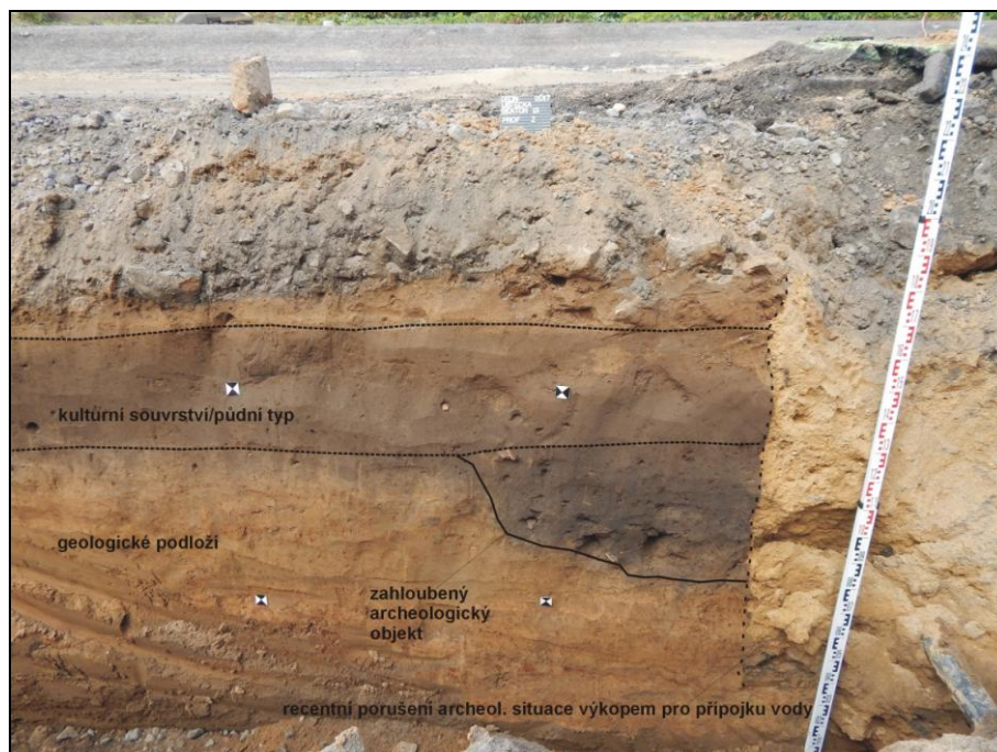
Obr. 02. Interpretovaný šikmý snímek pozitivní nálezové situace, opět porušený recentním zásahem (foto a kresba A. Káčerik).
